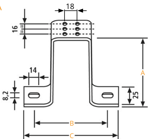
Typ A
