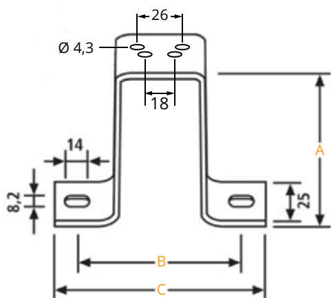
Typ D
